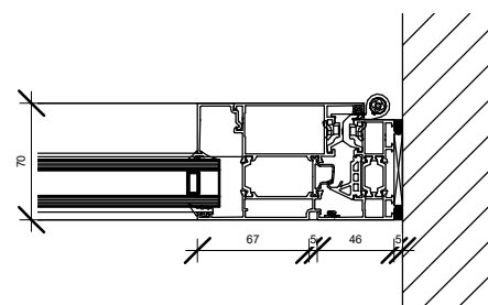
4 Detail 2 1 : 5
