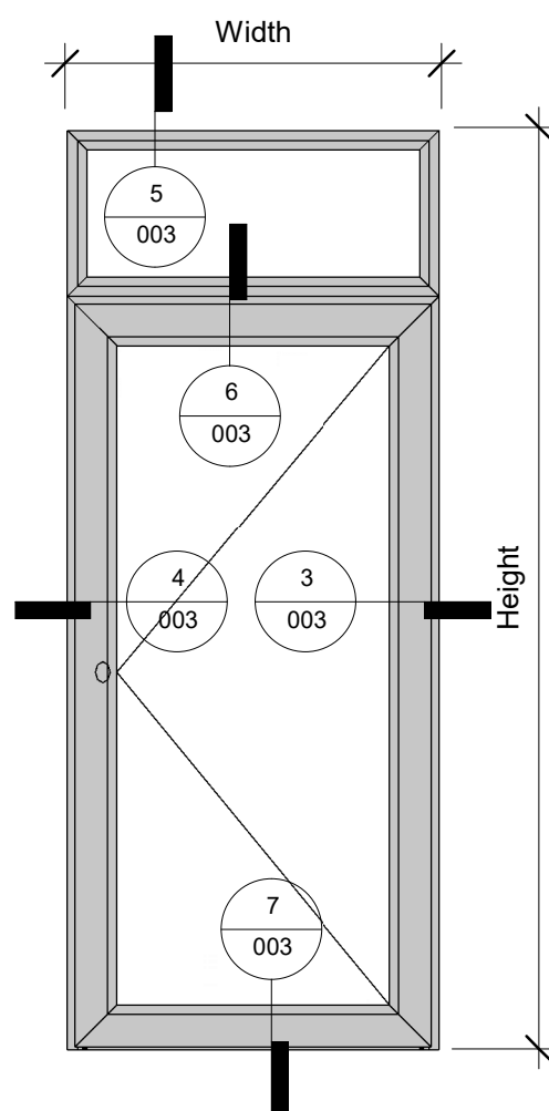
2 Elevation Back 1 : 20
