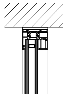
5 Detail 3 1 : 5
