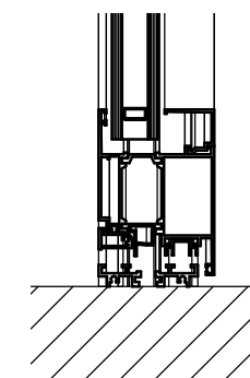
7 Detail 5 1 : 5
